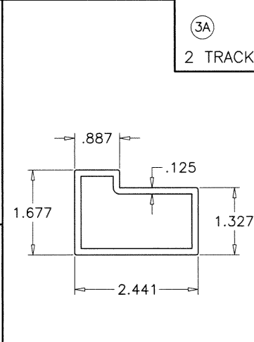
24 HOLLOW STIFFENER
