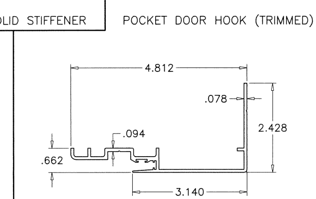
13 POCKET DOOR HOOK
