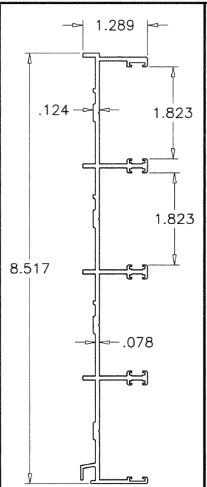
3C 4 TRACK FRAME JAMB
