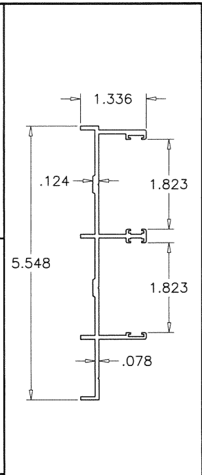
3A 2 TRACK FRAME JAMB
