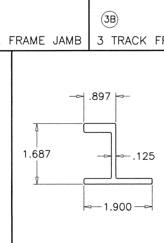
25 SOLID STIFFENER
