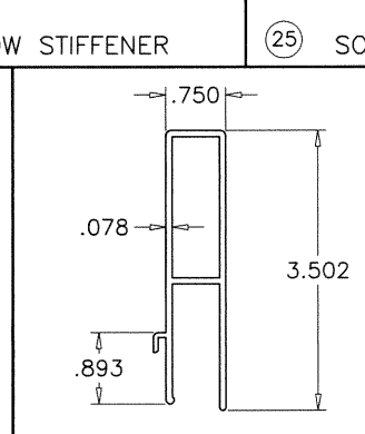
15B 3-1/2" SILL RISER
