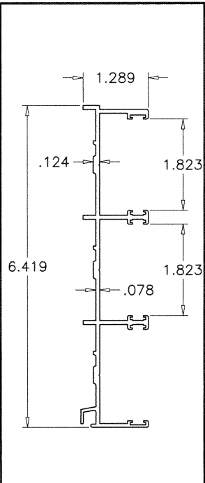
3B 3 TRACK FRAME JAMB
