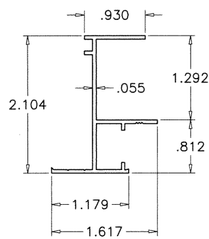
FRAME JAMB
